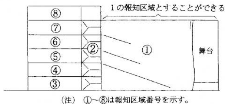
図14-1 吹き抜けがある場合の報知区域の設定例
