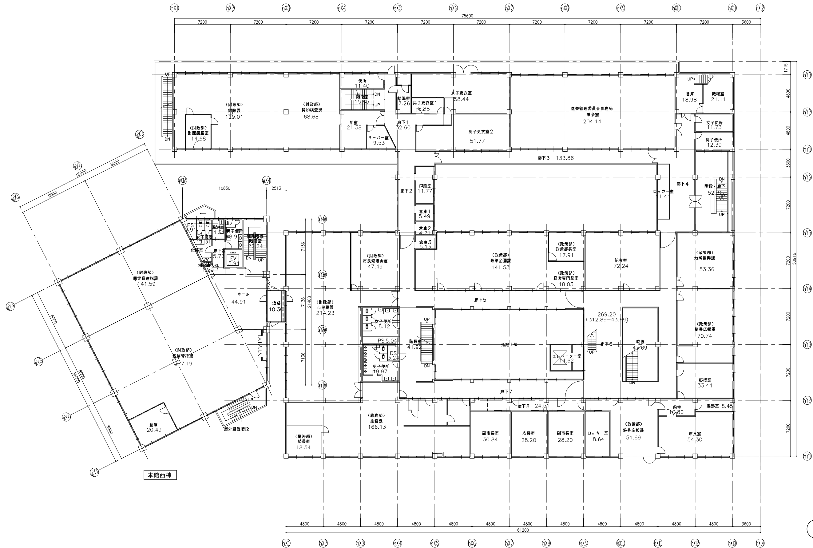
2階平面図 1/300
