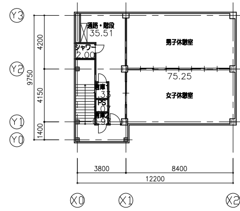
3階平面図 1/300
