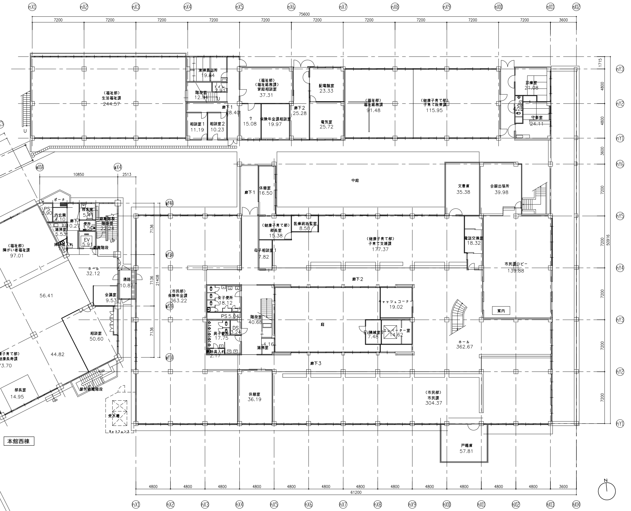
1階平面図 1/300
