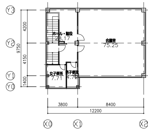
2階平面図 1/300
