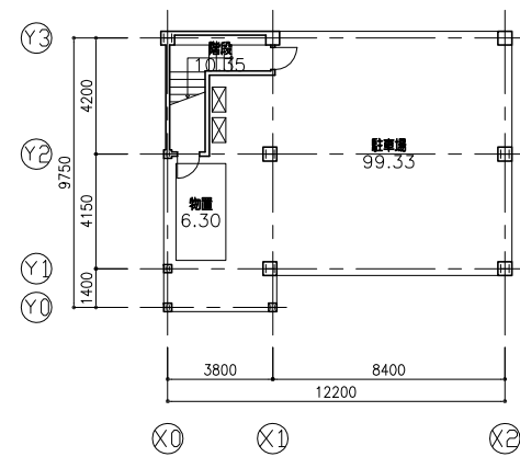
1階平面図 1/300
