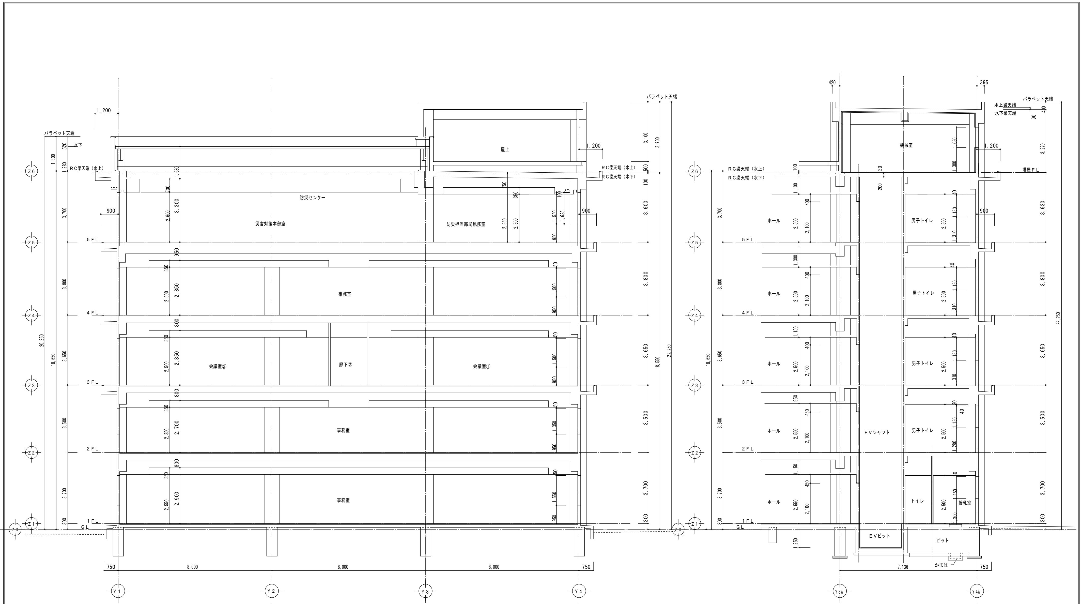
断面図 1:100
