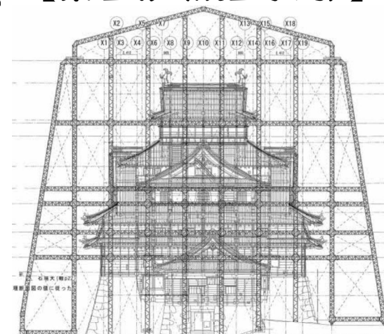
立面図(南面)
