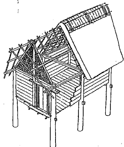
第225図 高床建築軸部構造模式図
