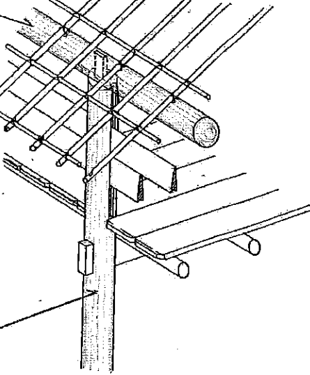
第225図 高床建築軸部構造模式図
