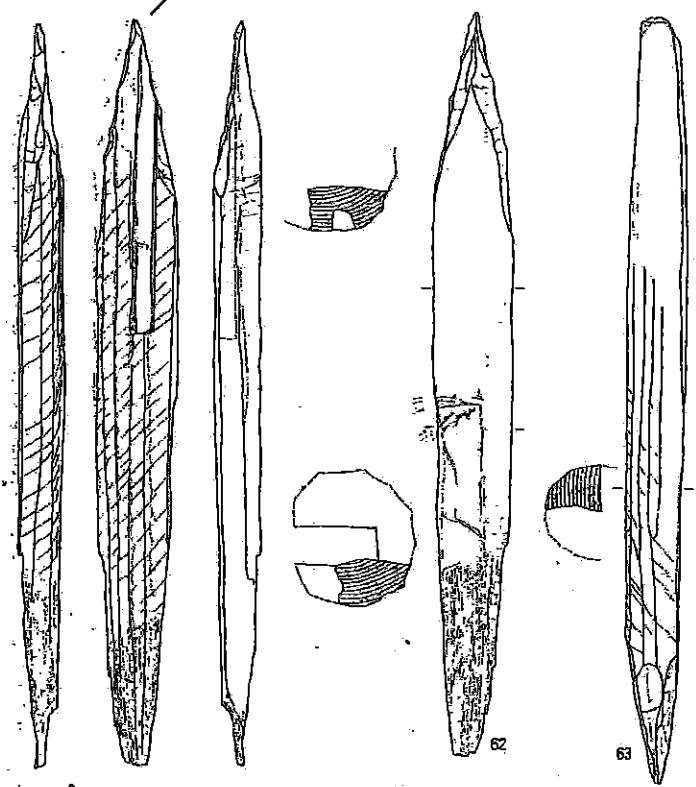
第65図 上小紋遺跡出土木器実測図
