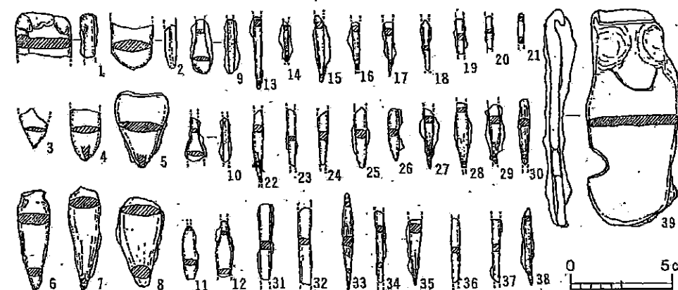
平所遺跡鉄製工具実測図
