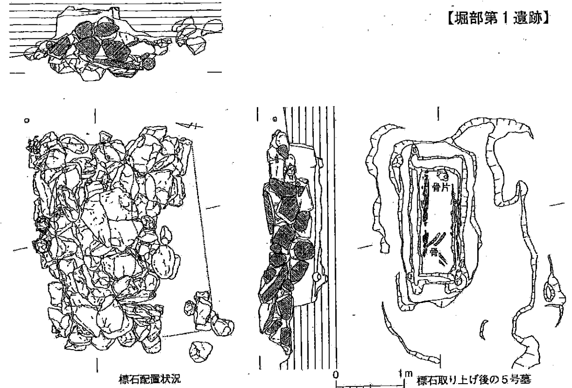
堀部第1遺跡5号墓実測図 (S=1:50)
