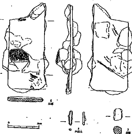
図16 上野II遺跡 板状鉄素材
