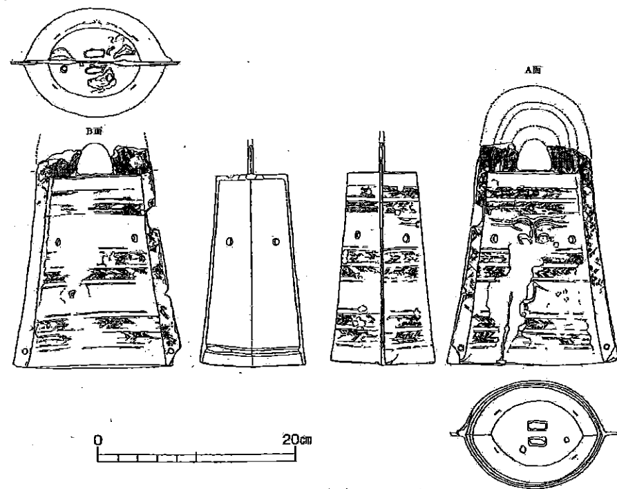
木橋家伝世銅鐸実測図 (S=1:5)
