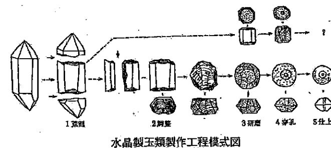
水晶製玉類製作工程模式図
