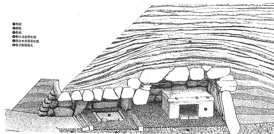
横穴式石室内部『史跡今市大念寺古墳保存修理工事報告書』出雲市教育委員会 1984
