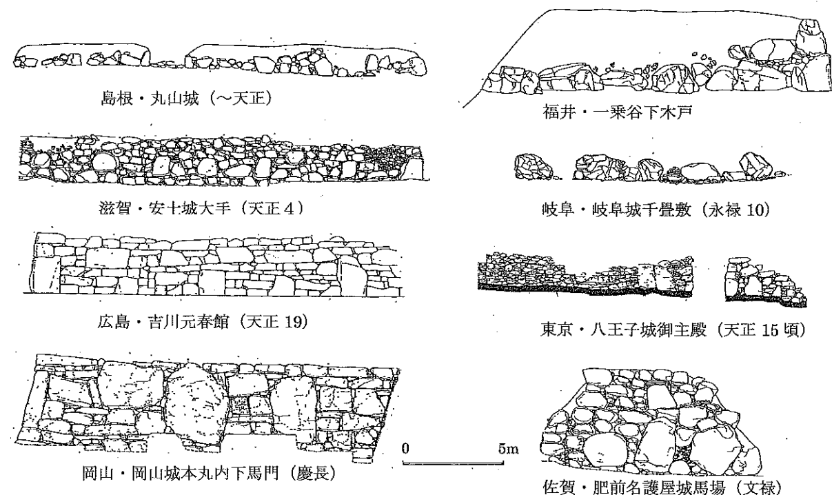
第7図 各地城の巨石・立石を組み込んだ門脇の石垣 各報告書などから作成
