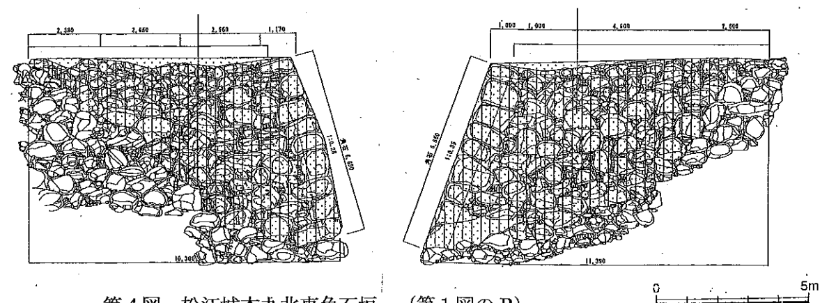
第4図 松江城本丸北東角石垣 (第1図のB) 松江市教育委員会 2007『松江城石垣修理報告書』から
