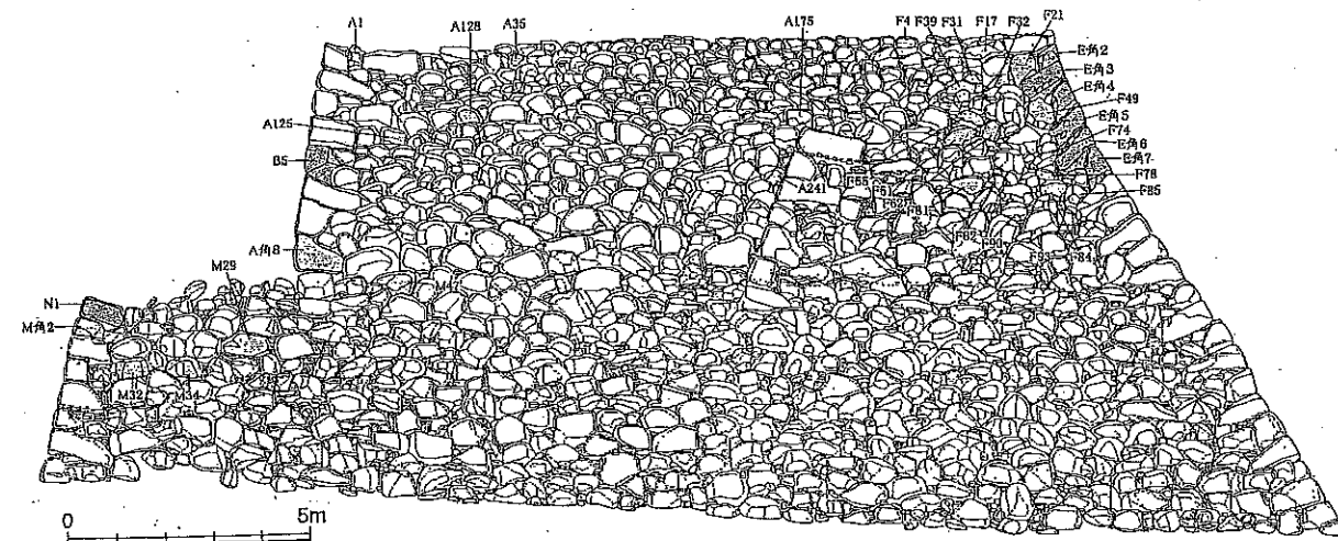
第6図 松江城腰曲輪東面石垣 松江市教育委員会 2007『松江城石垣修理報告書』から
