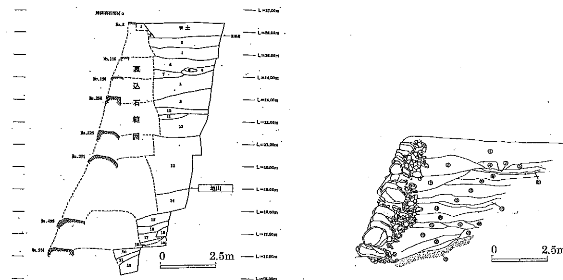
第5図 松江城本丸南東武具櫓石垣[左] (第1図K・L) と本丸北東角石垣[右] (同B) の断面 松江市教育委員会 2007『松江城石垣修理報告書』から
