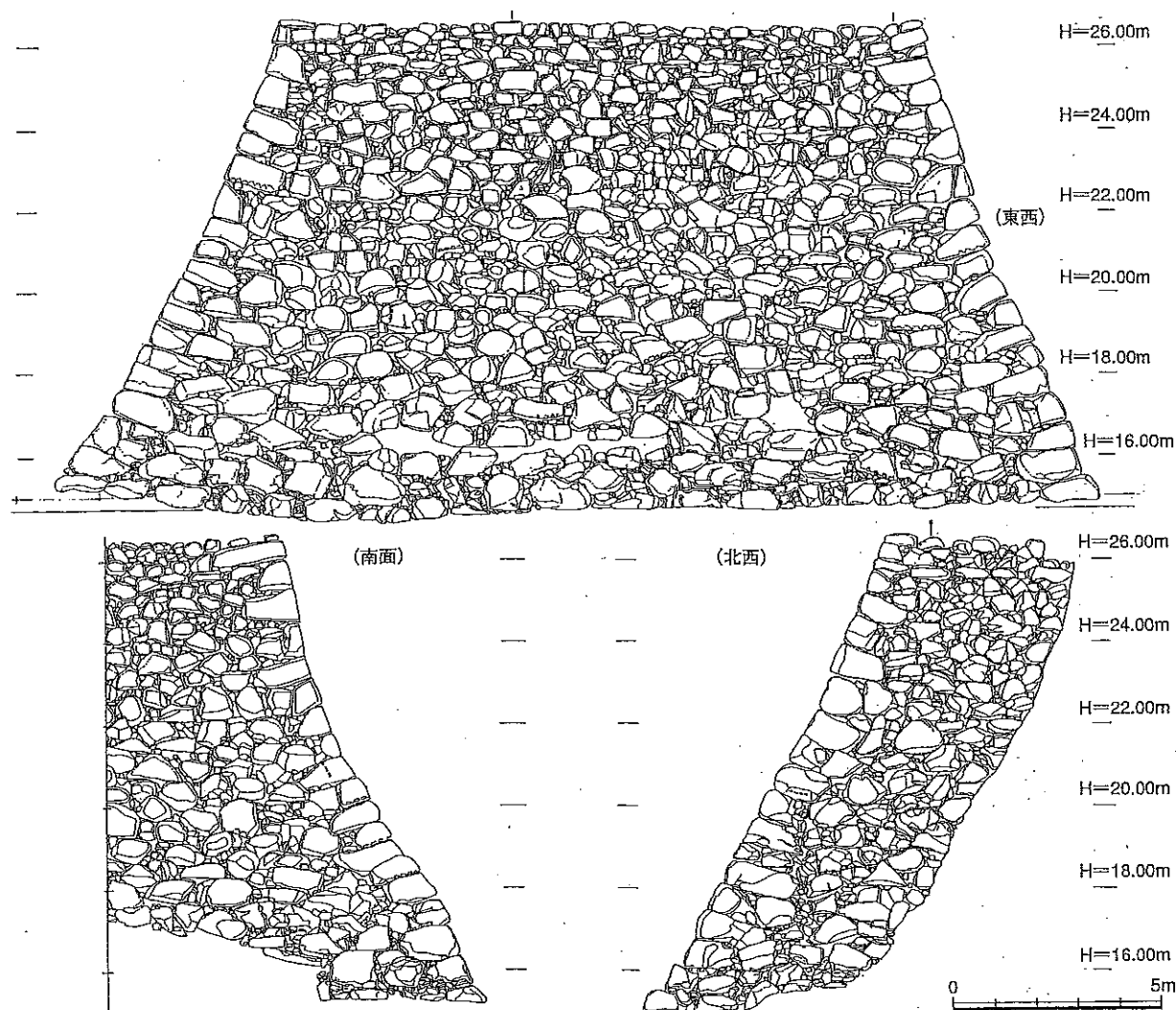
第3図 松江城本丸南東武具櫓の石垣 (第1図のK・L) 松江市教育委員会 2007『松江城石垣修理報告書』から
