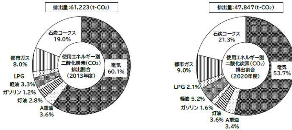
図6 二酸化炭素(CO 2 )排出比率(使用エネルギー別:2013年度・2020年度)
