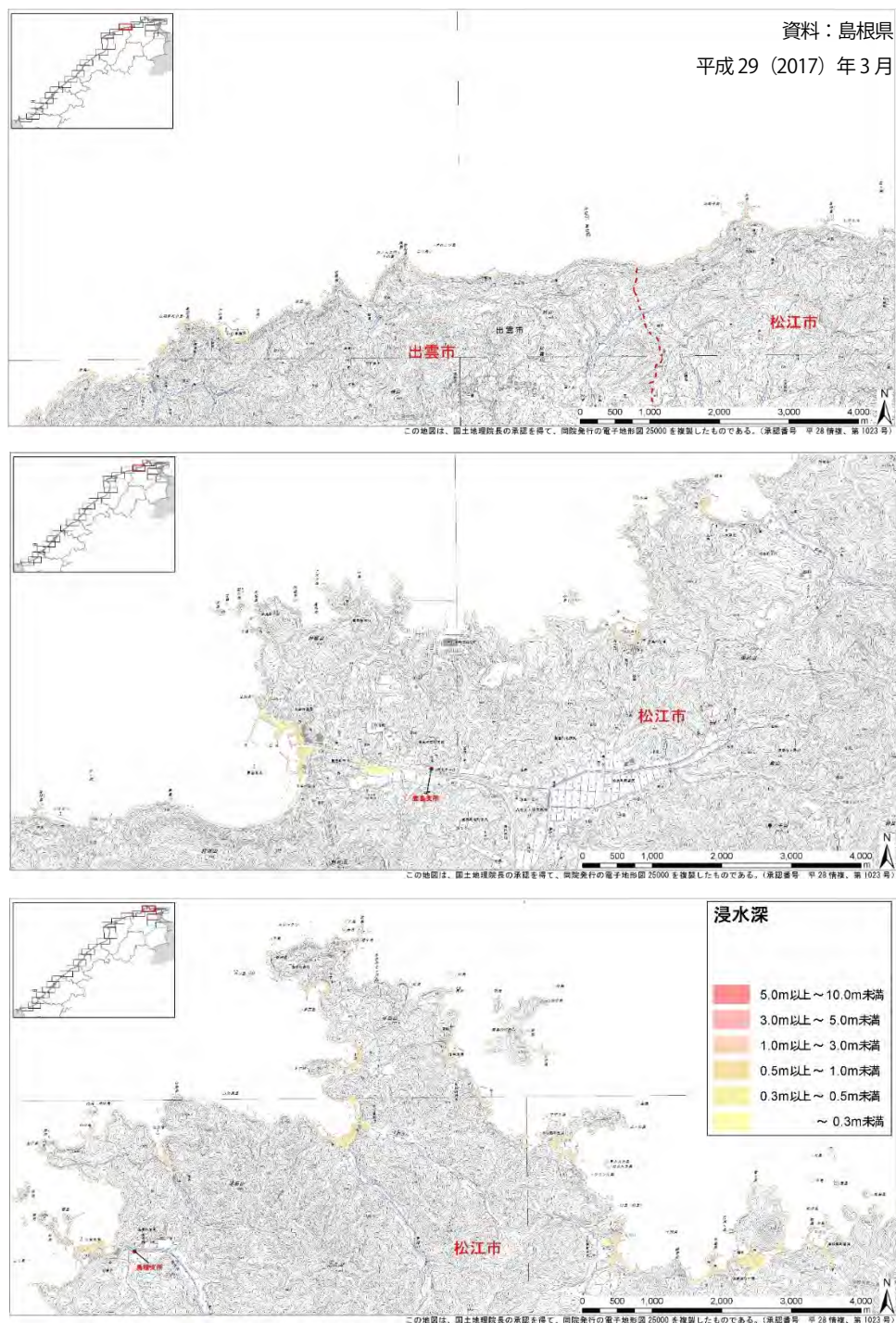
図 7-6 津波浸水想定区域(想定最大 L2)
