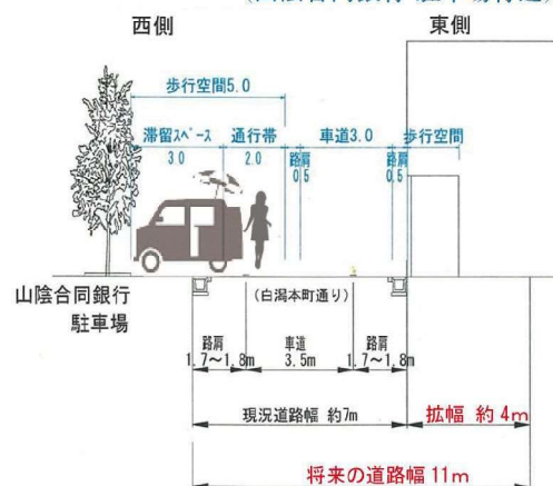
歩行者滞留空間 横断面図 (山陰合同銀行 駐車場付近)
