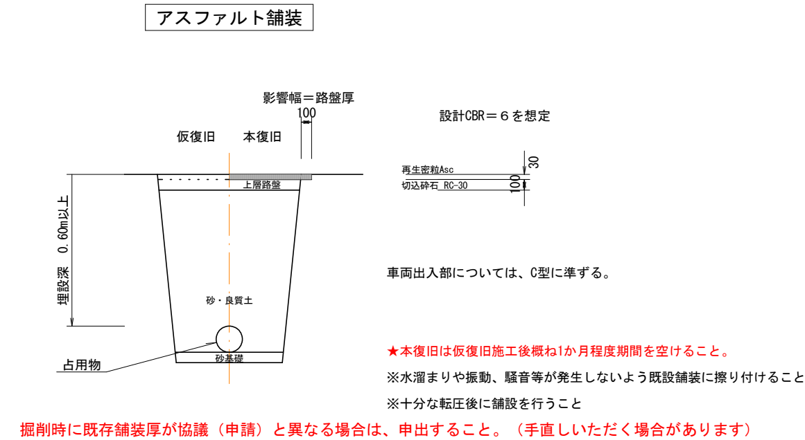
市道（歩道）掘削復旧標準断面図
